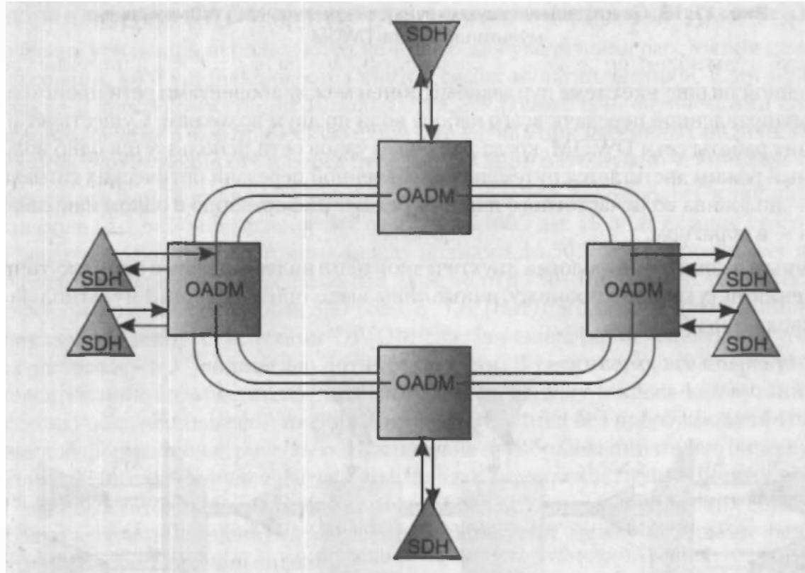
Кольцо мультиплексоров DWDM
